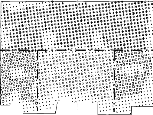
Abb. 4: Dachflächenanalyse (Verschneidungen, Sprünge)
